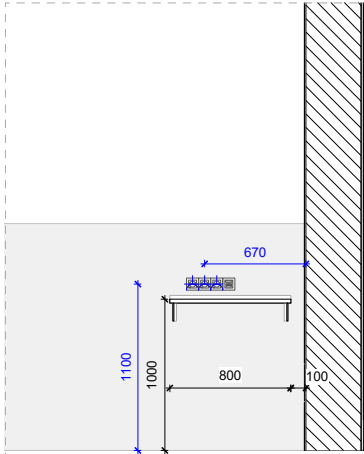
Ansicht 1 Lagerfläche Fahrzeughalle 1:50
