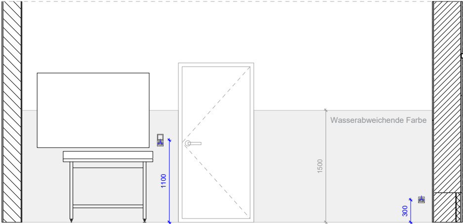
Ansicht 2 Lagerfläche Fahrzeughalle 1:50
