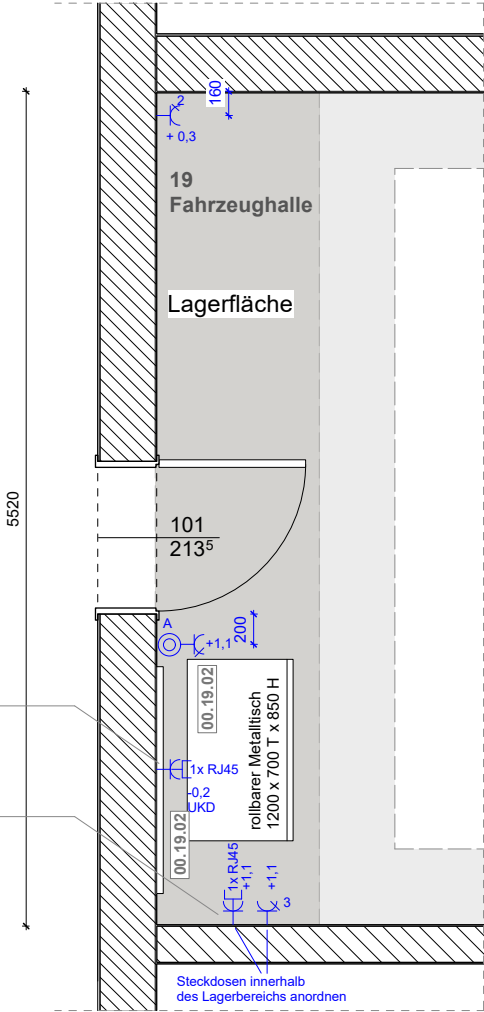
Grundriss Lagerfläche Fahrzeughalle 1:50
